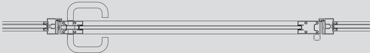
Sezione orizzontale della porta battente vetro con telaio "BIG". Horizontal section of hinged glass door with BIG frame
