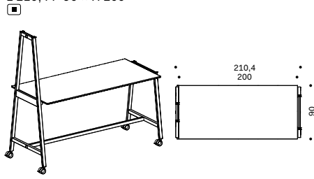
802MT0121_ Tavolo su ruote / Table on castors
